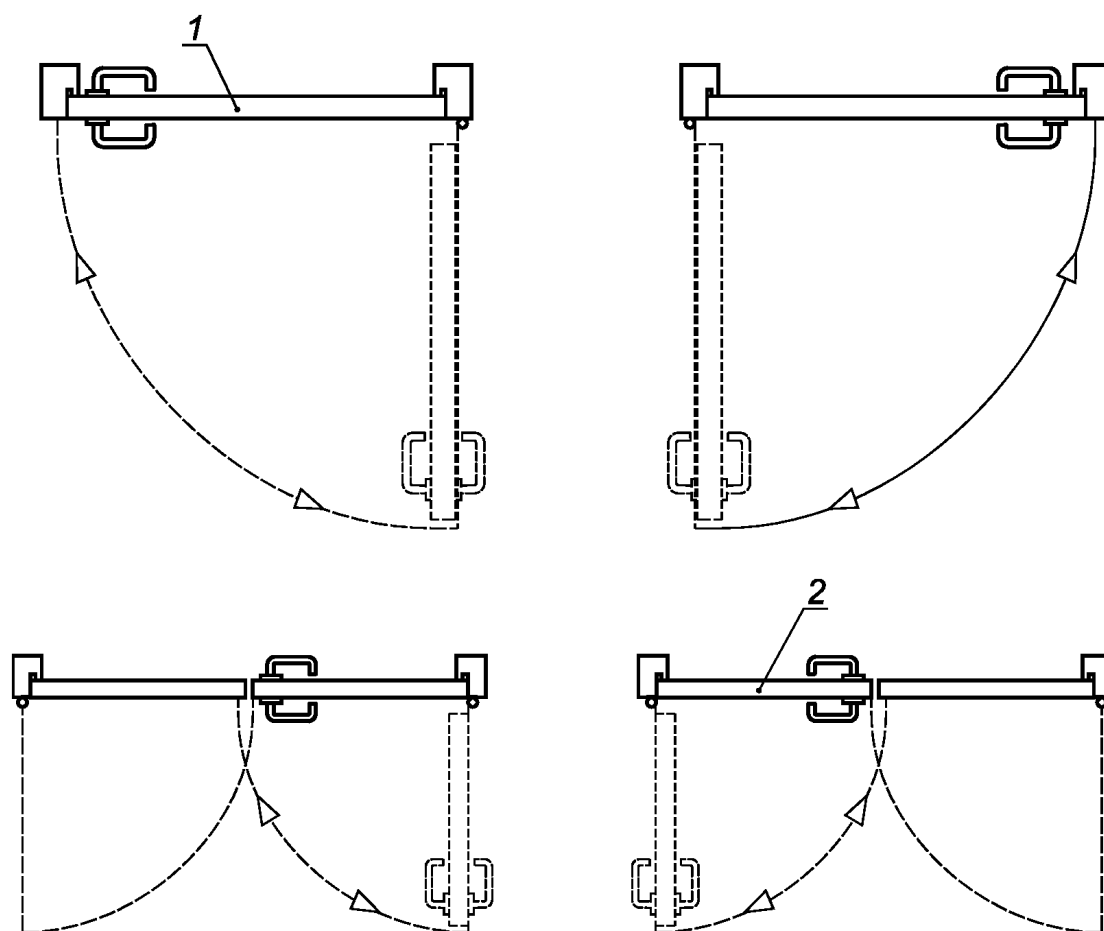
Рисунок А.3 — Примеры направления открывания дверей
