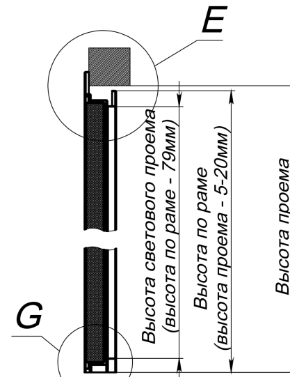
D-D (1 : 10)
