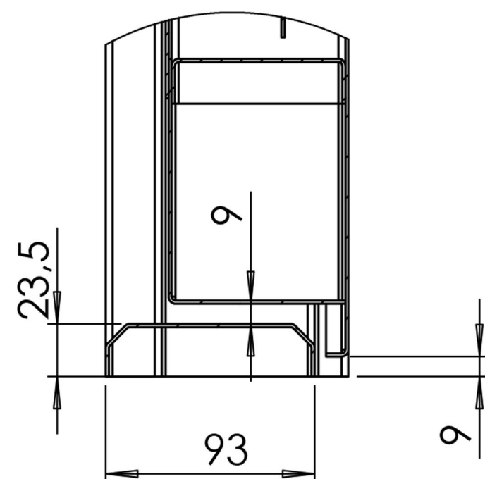
Порог 14 мм накатной МАСШТАБ 1 : 4
