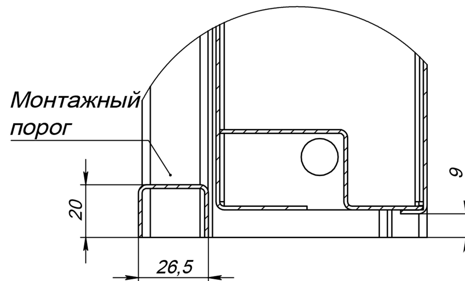
Автоматический врезной порог
