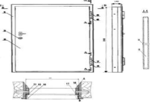
Рис. 1 Люк металлический
